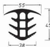
EP 45/55/38 (pro spáru 30)
