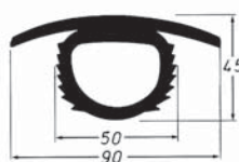
S 45/50/90 (pro spáru 30 - 40)
