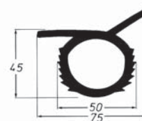
S 45/50/75 Eck (pro spáru 30 - 40)
