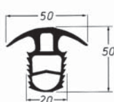
S 20/50 (pro spáru 20)
