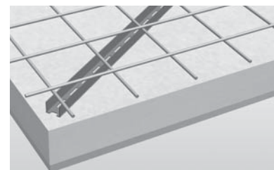
poloha D-lišty V na izolaci
